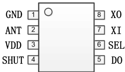
图3 WF510RA管脚排列图
