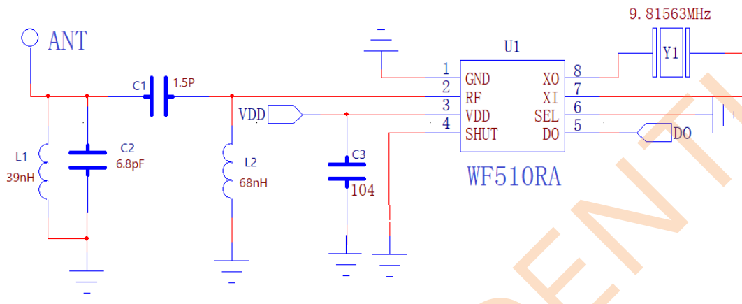
图1 315MHz 1.5kbps典型电路
