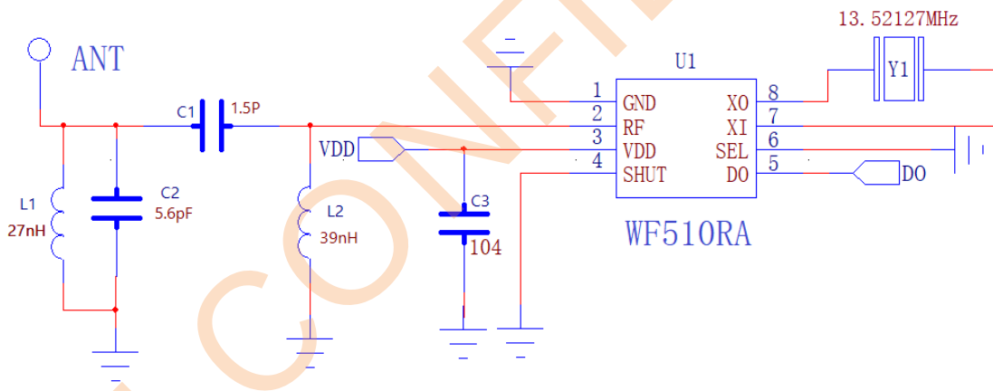
图2 433.92MHz 1.5kbps典型电路
