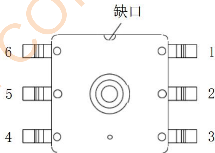
顶视图
