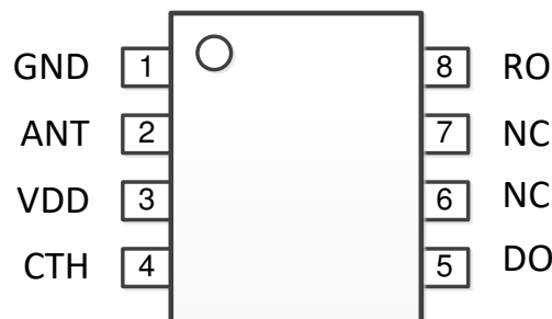
图3 WF550RA管脚排列图
