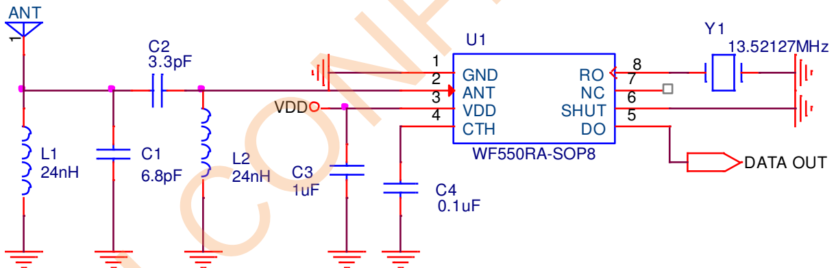
图2 433.92MHz 10kbps典型电路
