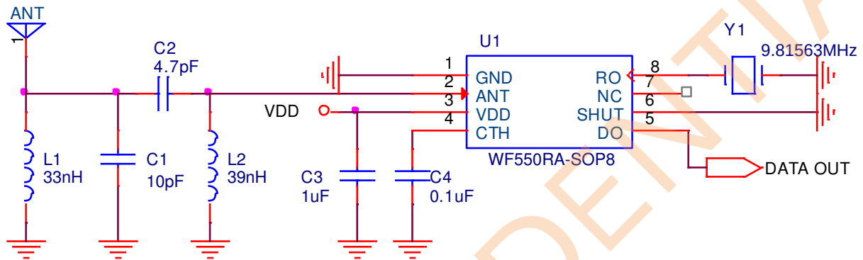
图1 315MHz 10kbps典型电路
