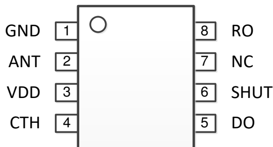
图3 WF490RA 管脚排列图
